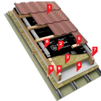
Рис. 6. Строение кровельной системы ТН-ЛЮКСАРД Мансарда
