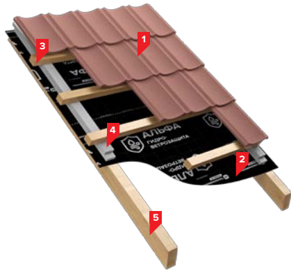
Рис. 5. Строение кровельной системы ТН-ЛЮКСАРД Классик
